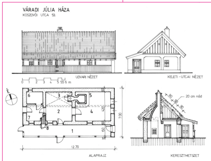
Háromsztatú parasztház. Zenta. Koszovói utca 53. Valkay Zoltán felmérési rajza, 1991.
