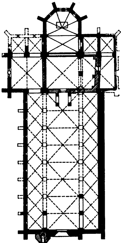
A monostortemplom izometrikus rekonstrukciója – a tetőszerkezet a 3. képen látható alaprajz szerinti állapotot ábrázolja
