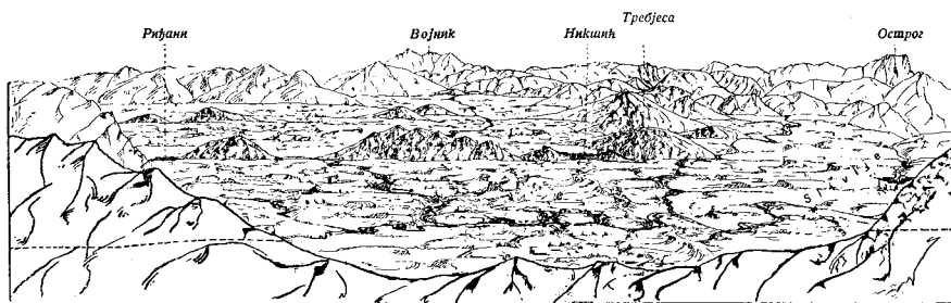
Никшићско карсно поље са хумовима (Црна Гора).
