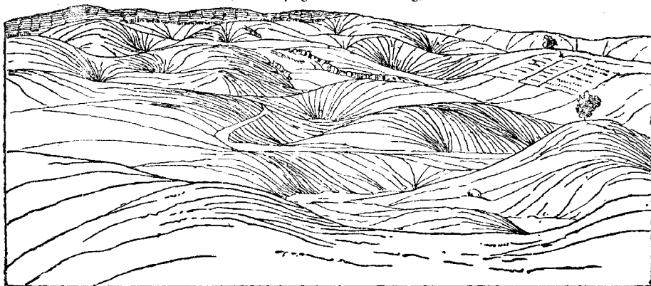
Мрежасни рељеф са вршачама у близини Карловца у Хрватској.
