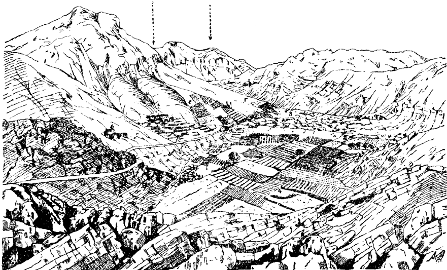
Обраћена увала Орахов До у Вали (Хумина у Херцеговини).
