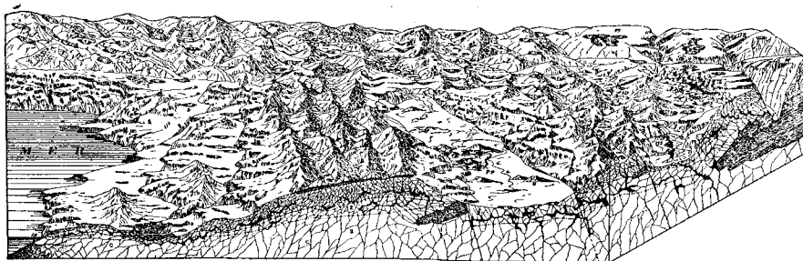
Шематска представа динарског карша.
