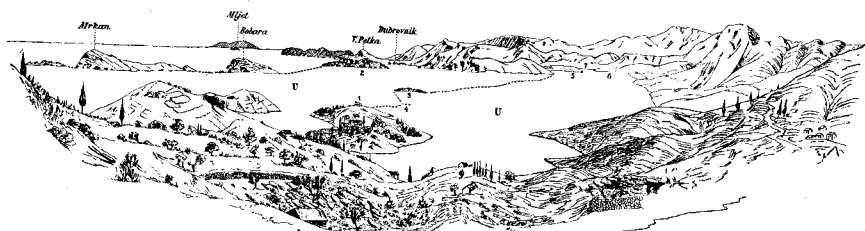
Низови увала (U), поштовани услед савишања и ушћаја абразије (Обала од Цавтата до Дубровника) 1 = Цавтат; 2 = клифови на Локруму, 3 и 4 = Супетак и Шуперка; 5, 6 и 7 = затони дубровачке жупе: Купари, Сребрно и Жупа.
