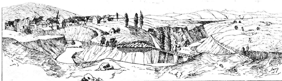
Насеља на старим стеновитим терасама (Слуњ на Корани у југозападној Хрватској)
