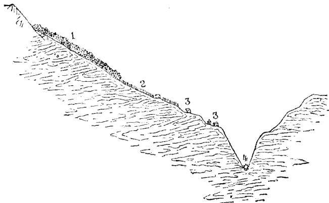
Села изнад Качаничке Клисуре (Стара Србија)
