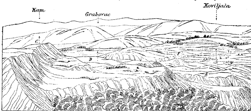
Чешири језерске терасе између Гучева и Ковиљаче код Лознице (C, D, E, F).
