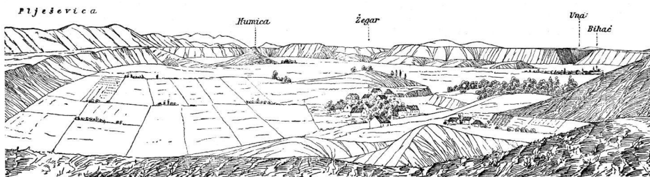
Бихаћска језерска котлина и терасе. (Западна Босна).
