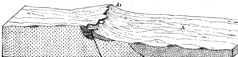
Шемашка представља језерске обале и површи.
