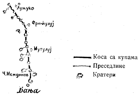
Еруптивне купе на Северу од Брестовачке Бање (Источна Србија)
