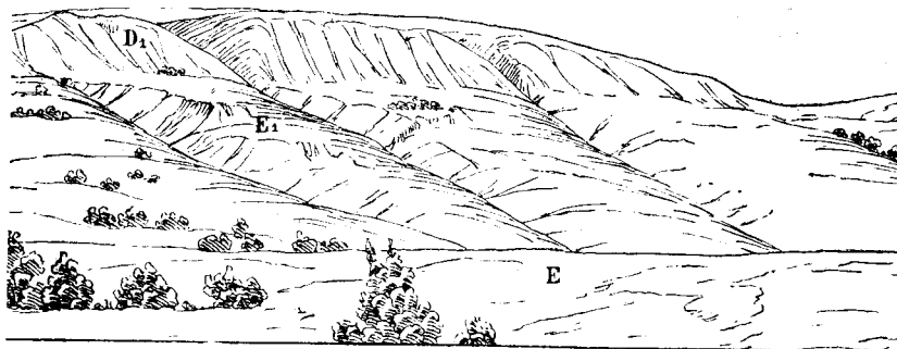
Клифови и обале на Пресеци код Орашца у Шумадији.
