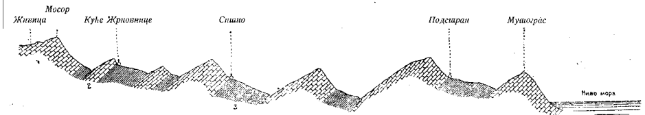
Насеља на геолошкој и морфолошкој граници. (Пољца под Мосором. Далмација) 1 = кречњак Мосора, 2 = кречњак уметнут у лапорима и глицима флиша; 3 = флиш.
