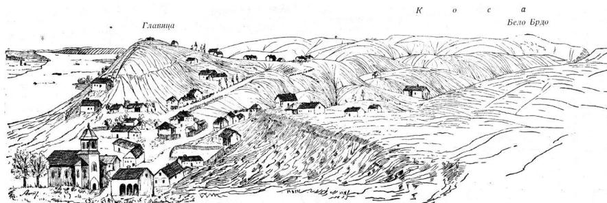
Присојни положај са уселинама (село Ритопек на Дунаву код Београда)
