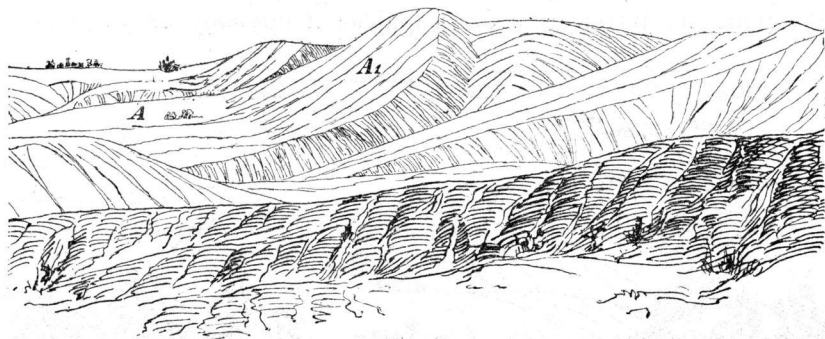
Речном челенком начеша језерска обала (код Чајетине у југозападној Србији).
