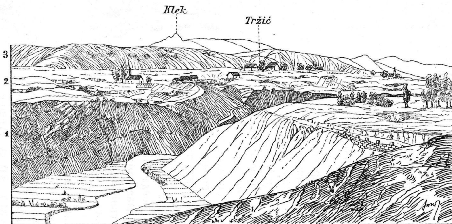
Насеља на флувијалној површи Мрежнице у југозападној Хрватској. 1 = флувијална површина; 2 = флувијална површина на којој насеља.
