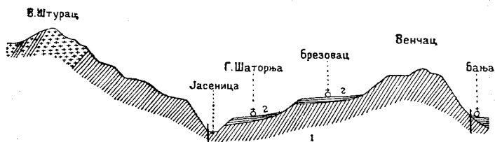
Профил кроз језерске површи Рудника и Венчаца.
