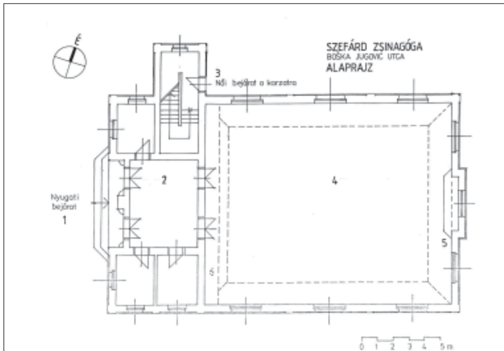
91. A „kis zsinagóga” alaprajza
